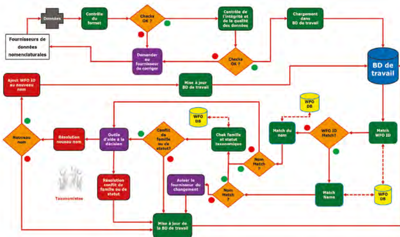
Workflow du fournisseur à la mise à jour du référentiel taxonomique de la WFO que devra gérer Botalista.
